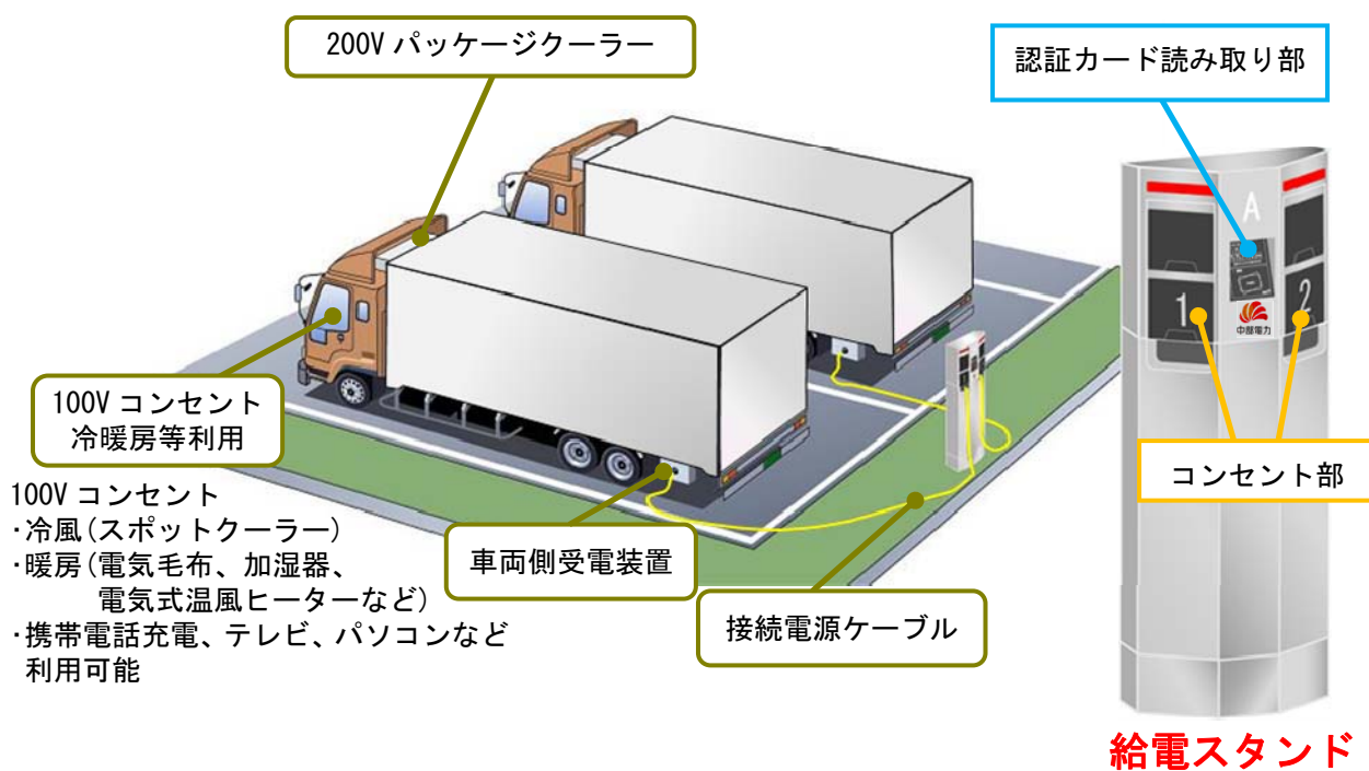
外部電源式アイドリングストップ給電システムのイメージ図
