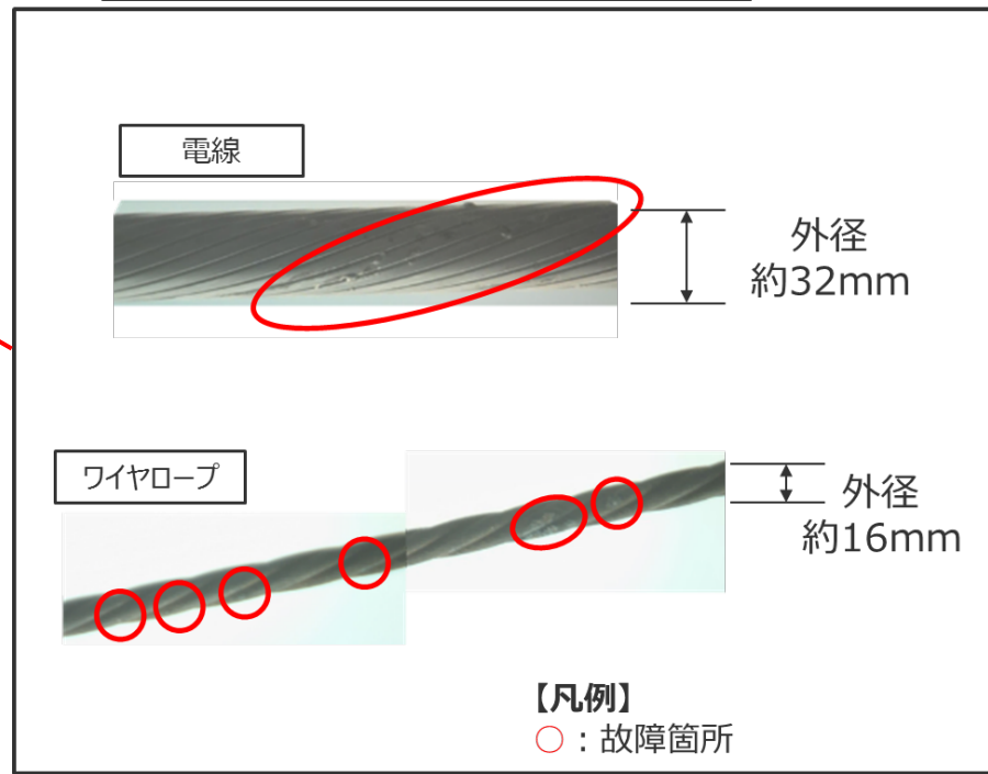
故障箇所の電線とワイヤロープ (写真)
