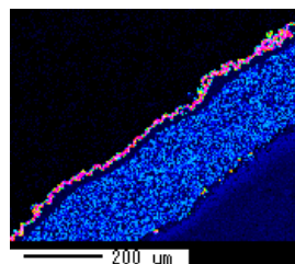
【火力】ガスタービン動翼の遮熱コーティング分析例
