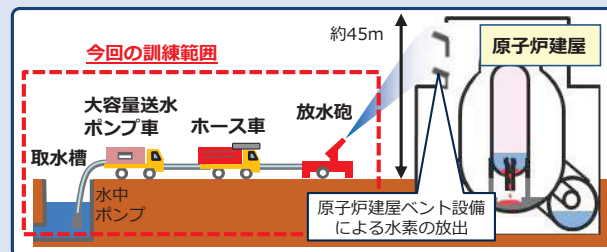
拡散抑制設備（大容量送水ポンプ）使用イメージ図
