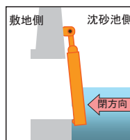
排水用フラップゲートの原理
