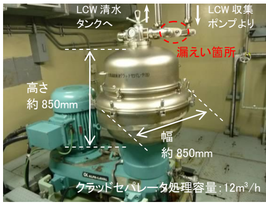
クラッドセパレータ(B)外観
