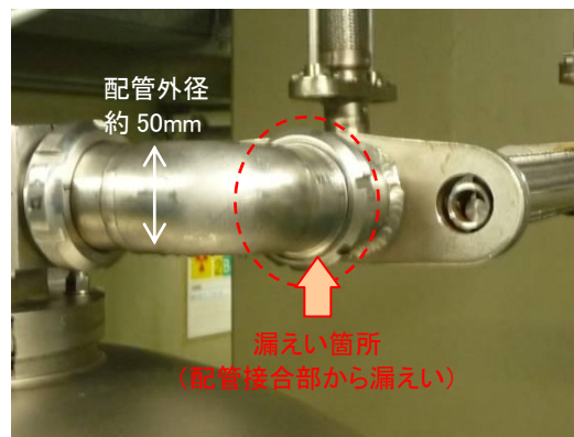
クラッドセパレータ(B)入口配管 漏えい箇所の拡大写真(漏えい停止後)
