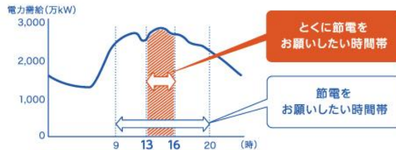
夏の平日の電気の使われ方(注)
