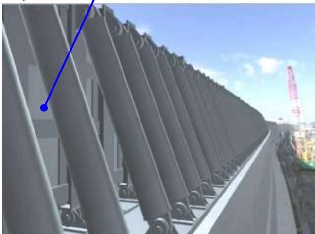
＜一般部・放水路部嵩上げイメージ図＞
