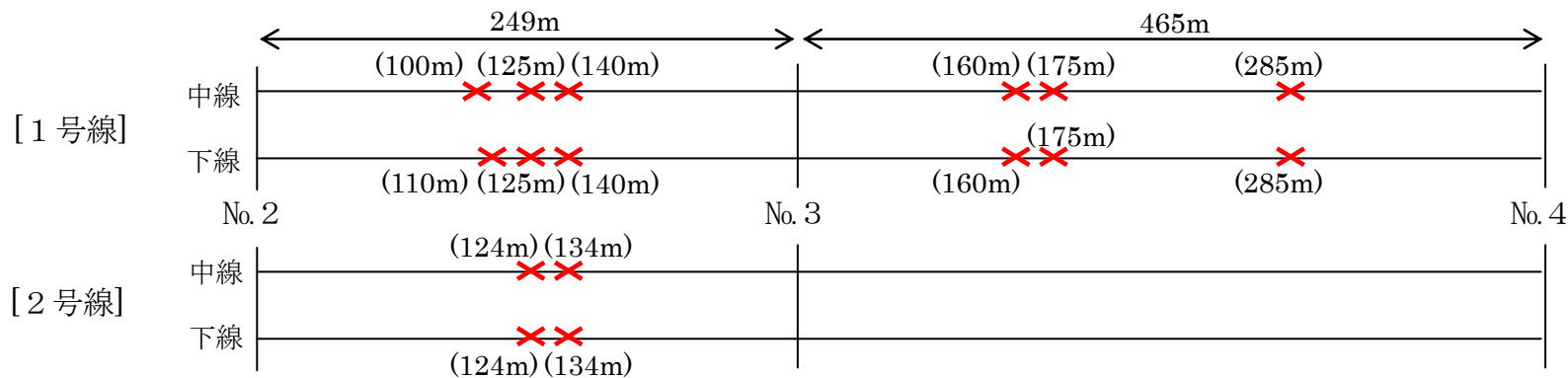
図1 現地確認された故障点
