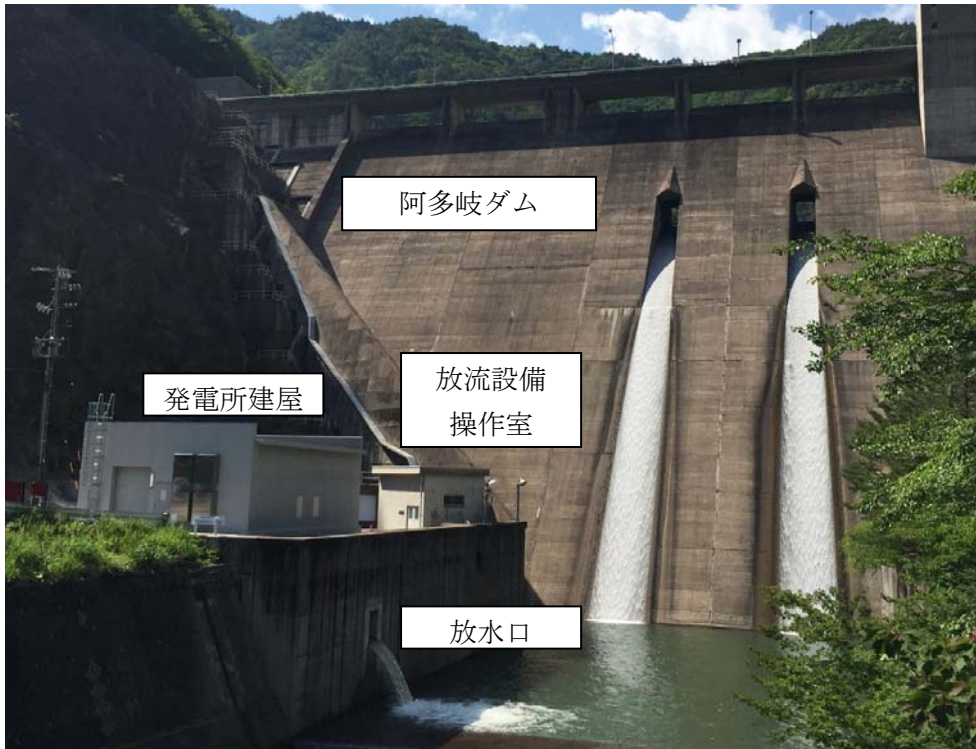
阿多岐発電所全景
