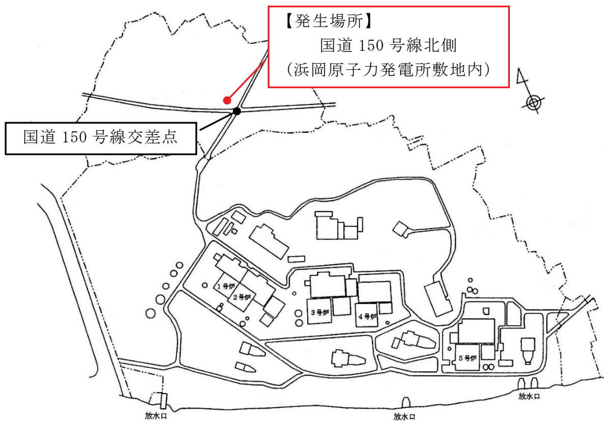
火災発生場所（発電所敷地図）
