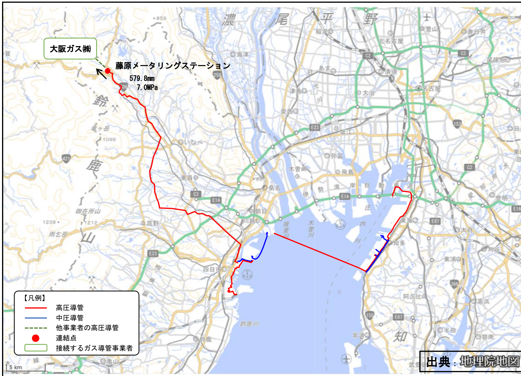
第8表 主要導管図
