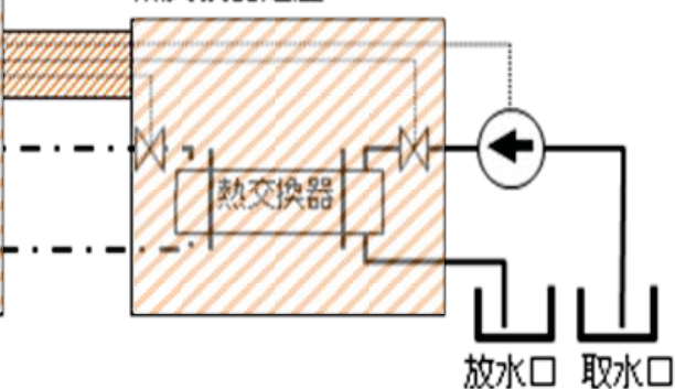
系統概略図(浜岡4号機の例)
