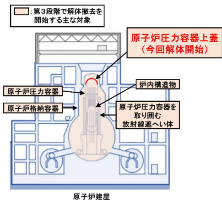
廃止措置第 3 段階の主な解体範囲
