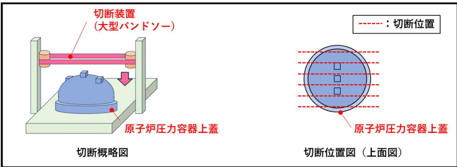
原子炉圧力容器上蓋切断のイメージ図
