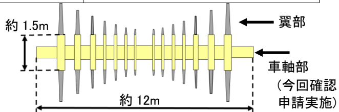
タービンロータのイメージ図
