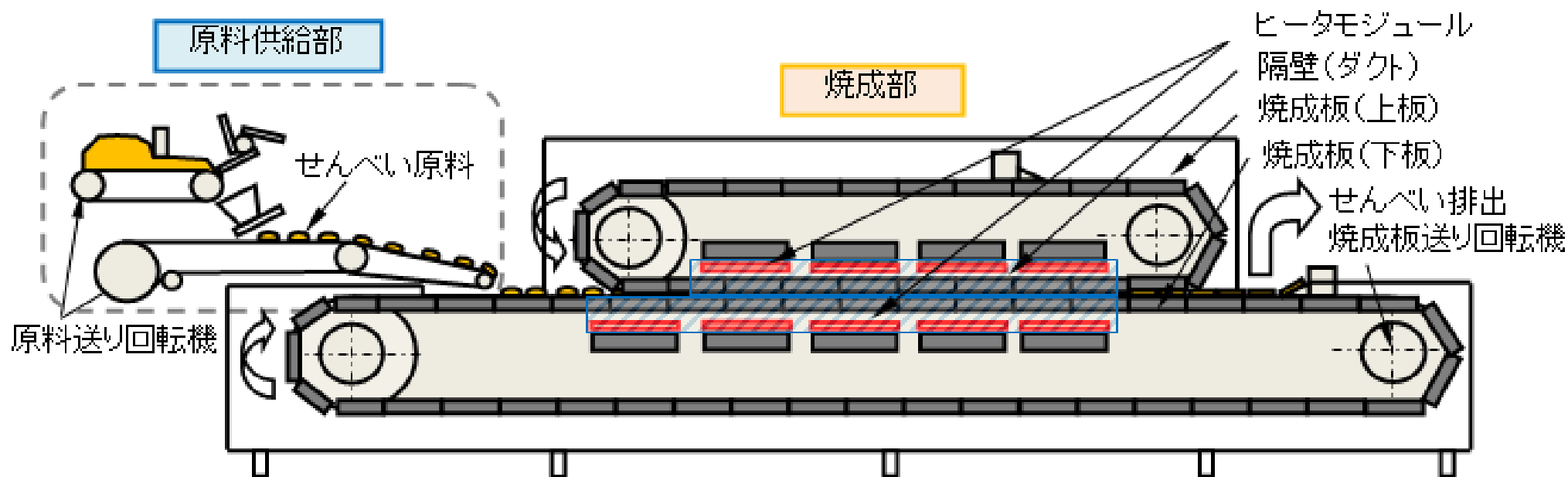
第3図 電気式焼成機の構成図
