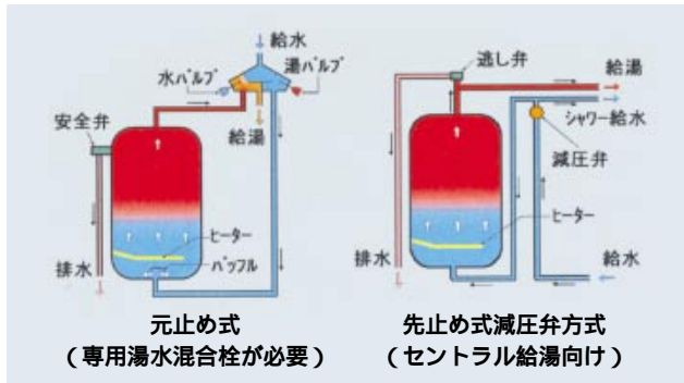
第1図 温水器の基本構造
