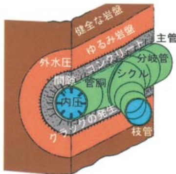
第1図 奥美濃発電所水圧鉄管分岐管の岩盤負担の概念
