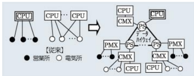
第2図 総合パケット交換網
