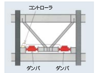
第4図 ダンパ取付図
