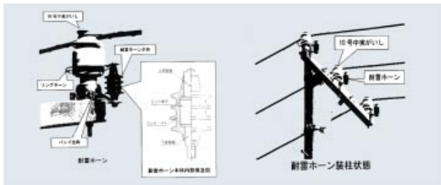
第1図 耐雷ホーン
