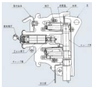
第2図 耐雷PC
