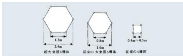
第1図 導体構成の比較
