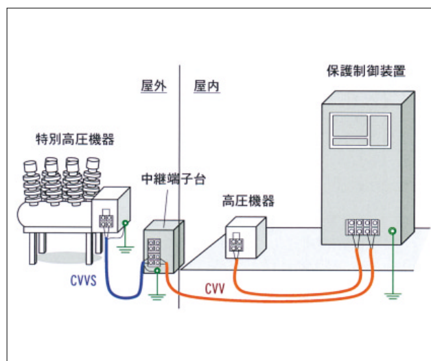
第5図 サージ電圧の抑制事例
