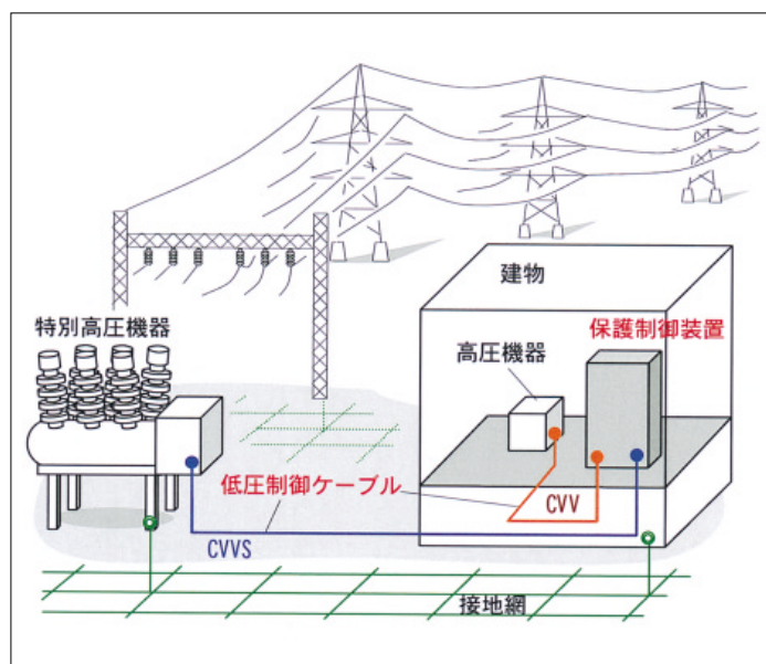
第1図 変電所における低圧制御回路の構成
