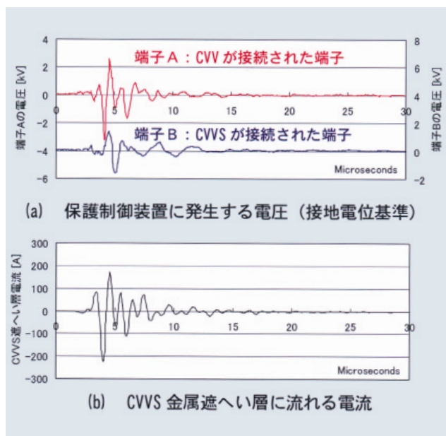
第3図 落雷時に保護制御装置に発生するサージ
