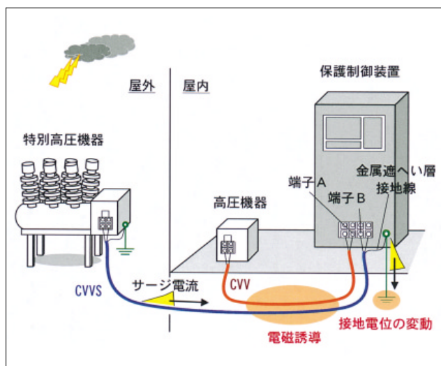
第4図 サージの侵入ルート・サージ電圧の発生機構
