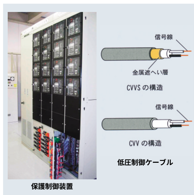
第2図 保護制御装置および低圧制御ケーブルの外観
