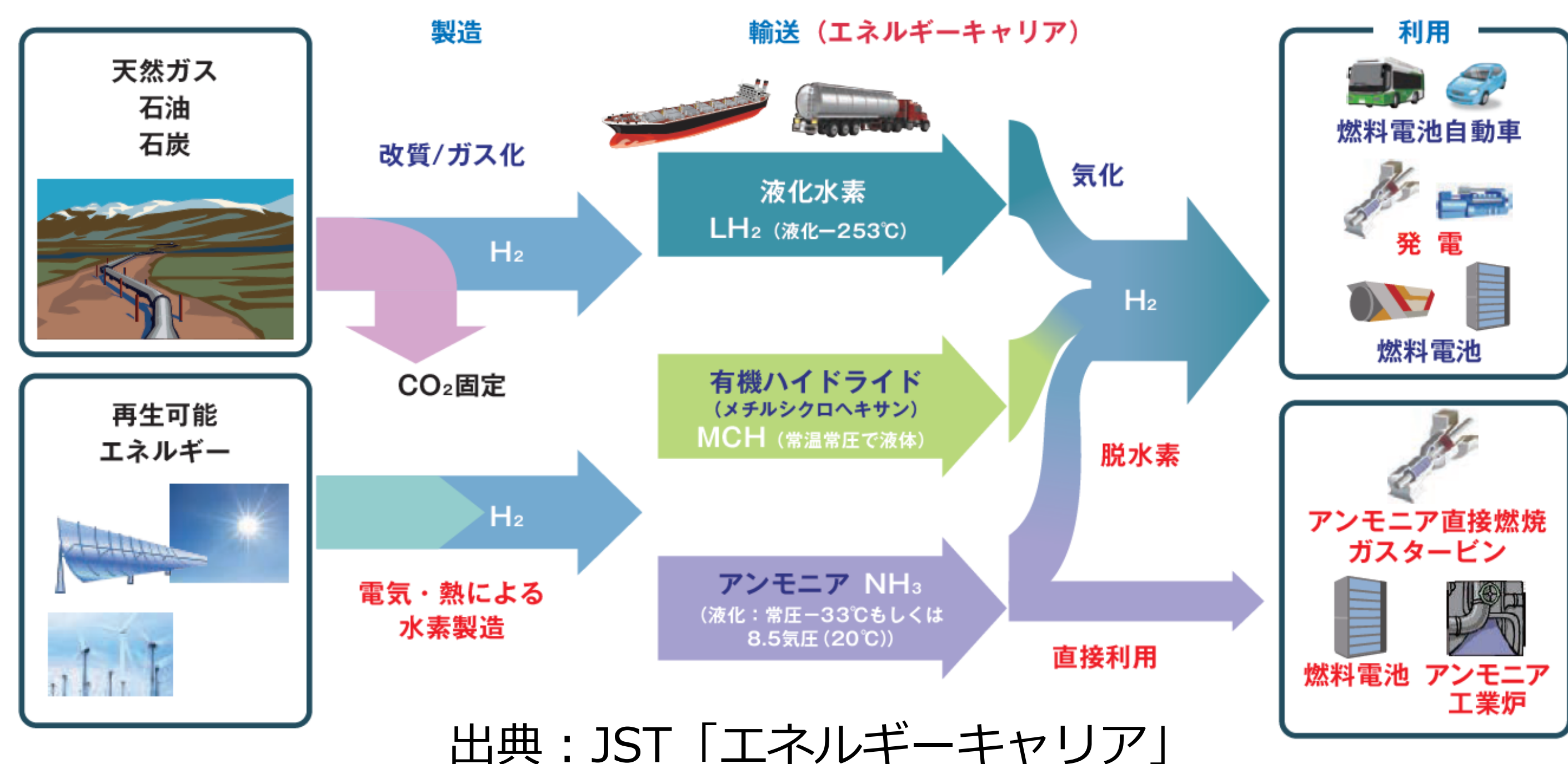
エネルギーキャリアの取組み〈CO 2 フリー水素バリューチェーンの構築〉
