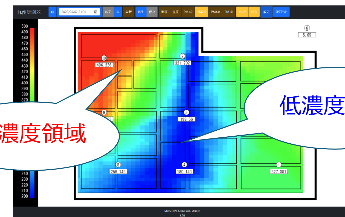
工場内オイルミスト濃度分布画面
