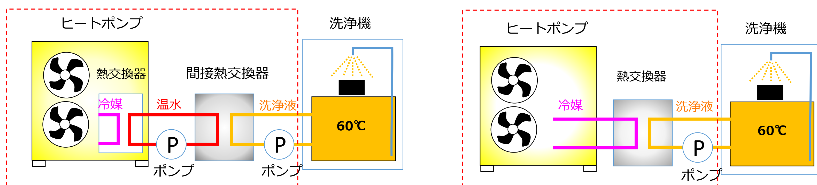
従来HPシステム（間接加温）
