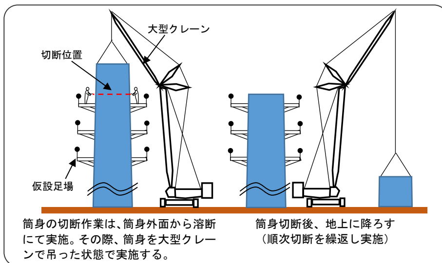
筒身の切断方法(イメージ図)
