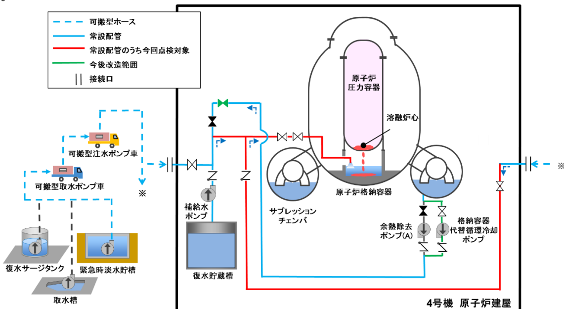
原子炉格納容器下部注水系統 概要図
