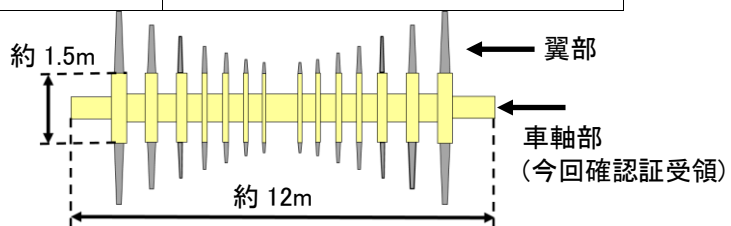
タービンロータのイメージ図
