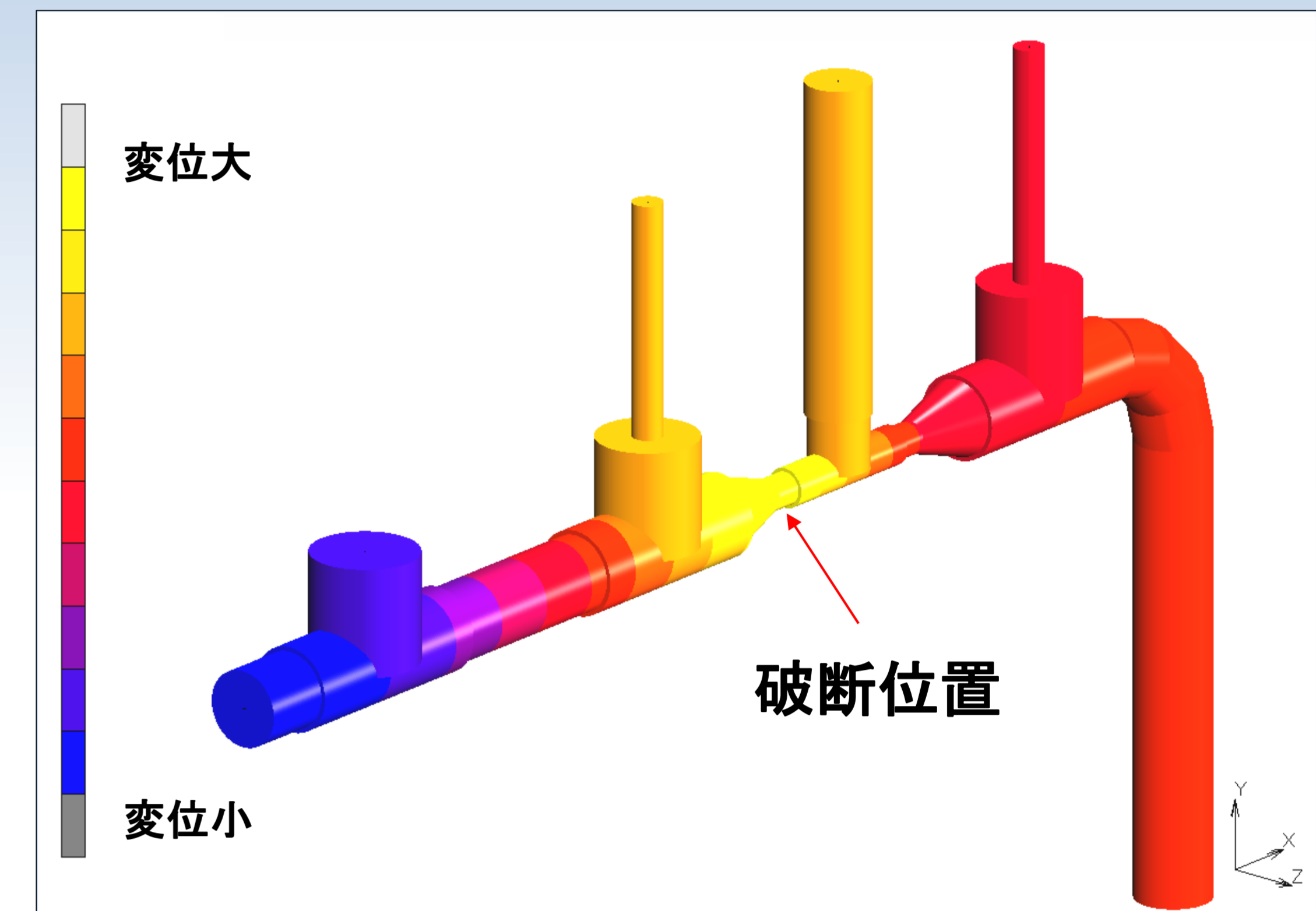
配管振動時の変位分布の例
